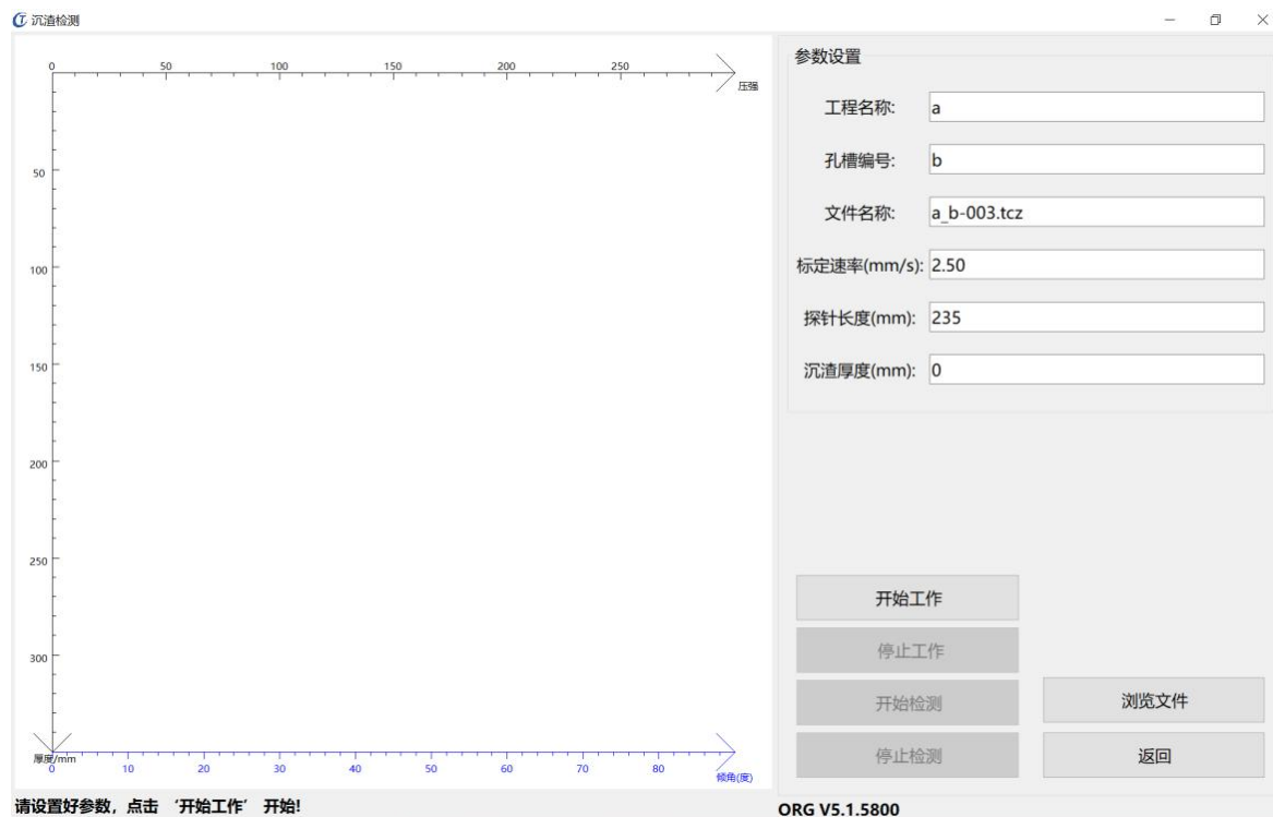
图3-20 沉渣检测
