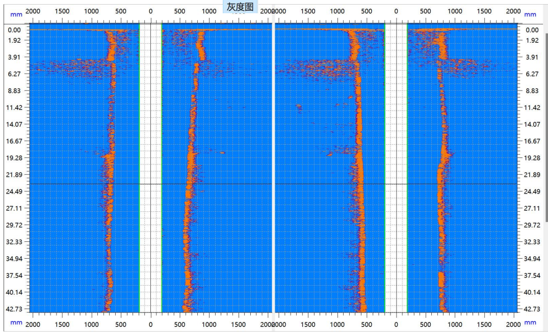
图4-11 灰度图
