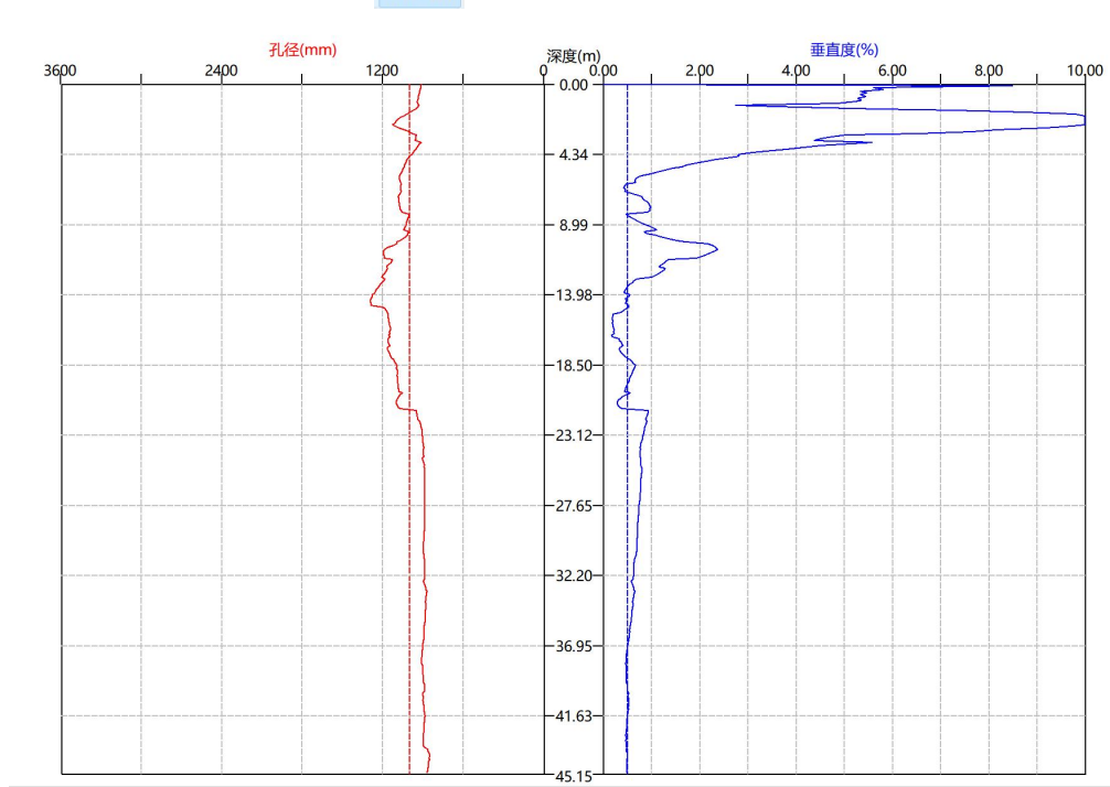
图4-13 HDV图
