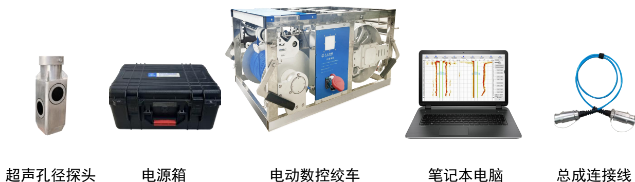
图1-1 型号示意图
