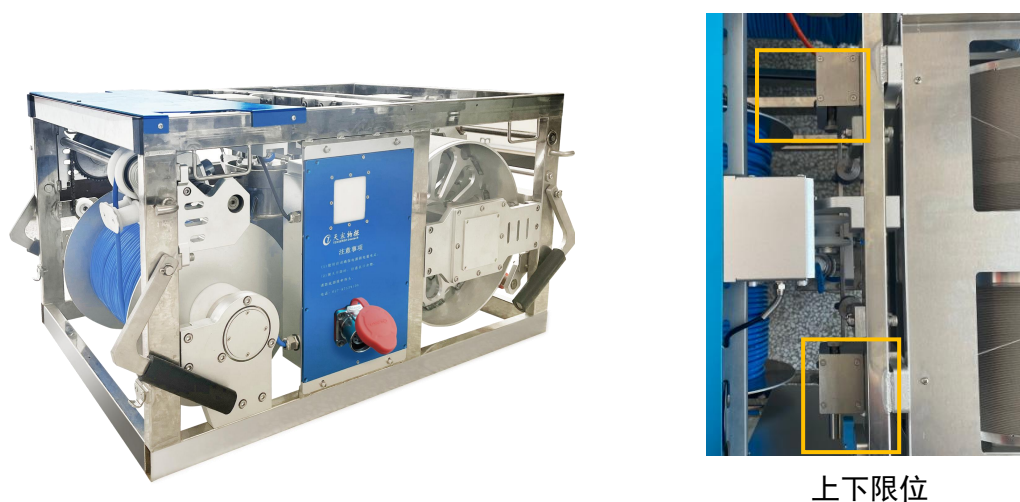
图1-2 绞车示意图
