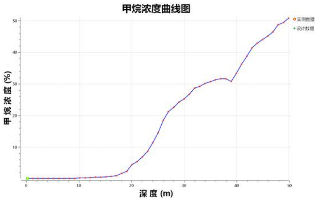
钻孔沿程甲烷浓度曲线图
