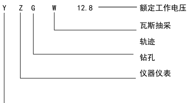
图1-1 型号示意图
