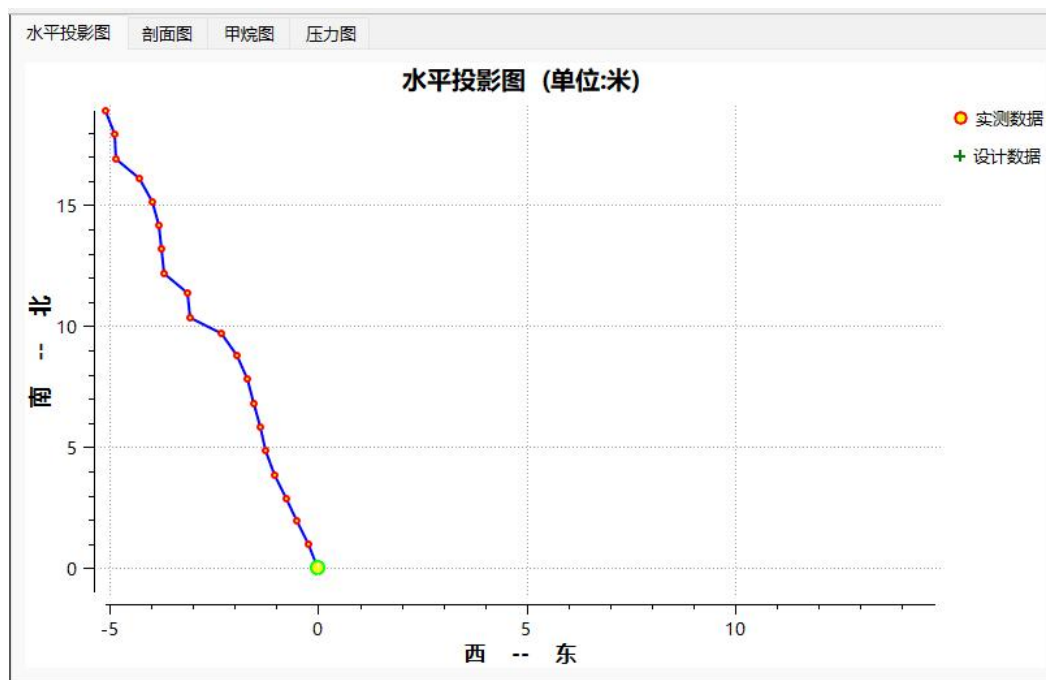
图3-13 查看视图
