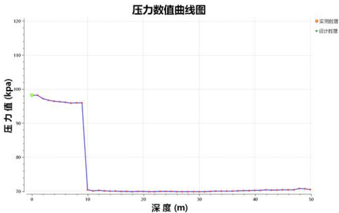
钻孔沿程抽采负压曲线图
