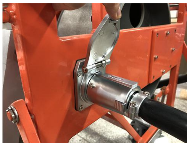
图1-7 连接14芯绞车航插
