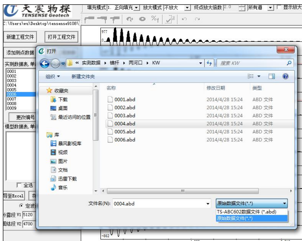
图 4-2 新建工程
