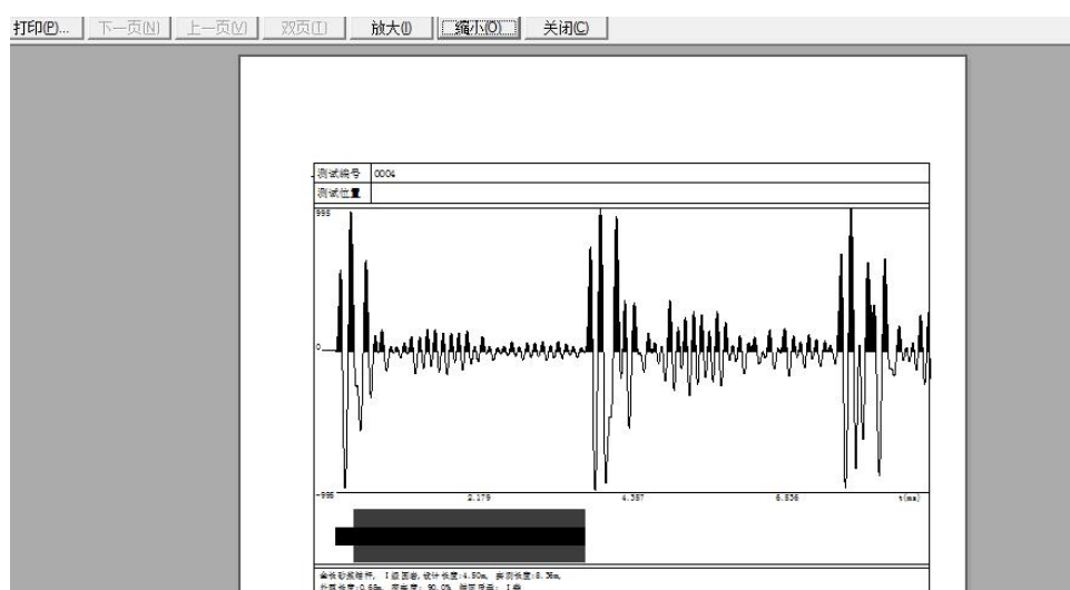
图 4-4 打印预览
